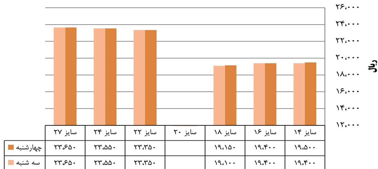
نمودار قیمت تیر آهن-ذوب آهن-اصفهان
